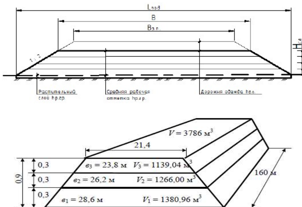
Рисунок 4 – Расчетная схема к определению послойных объемов земляных работ
